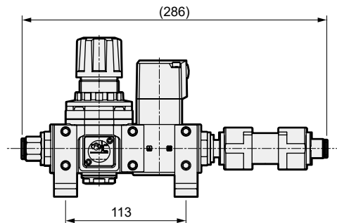
●CAU30-□-R□V□F (레귤레이터, 밸브, 필터)
