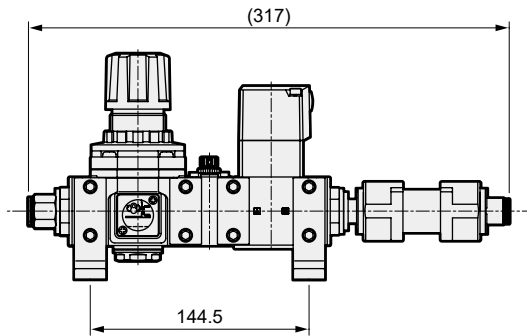
●CAU30-□-R□N1V□F (레귤레이터, 니들, 밸브, 필터)
