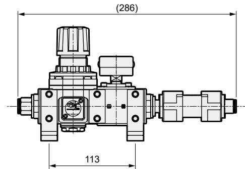
●CAU30-□-R□F (레귤레이터, 필터)
