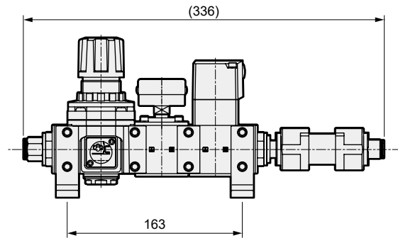
●CAU30-□-R□GY49V□F (레귤레이터, 압력계, 밸브, 필터)
