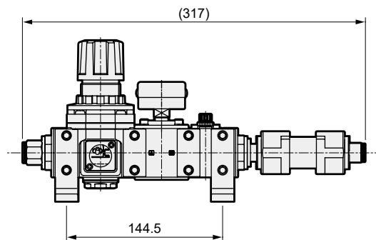
●CAU30-□-R□V□F (레귤레이터, 밸브, 필터)
