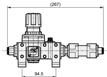
●CAU30-□-R□N1F (레귤레이터, 니들, 필터)
