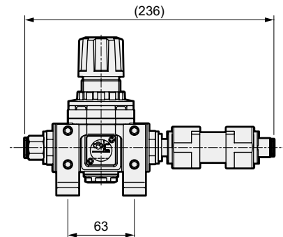
●CAU30-□-R□F (레귤레이터, 필터)
